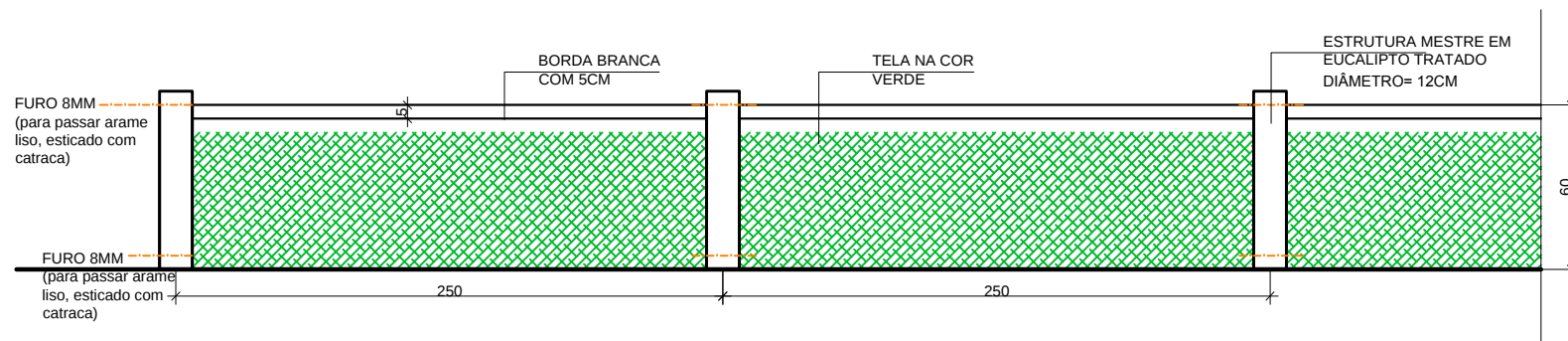
DETALHE CERCA DE PROTEÇÃO ESC..... 1/20
